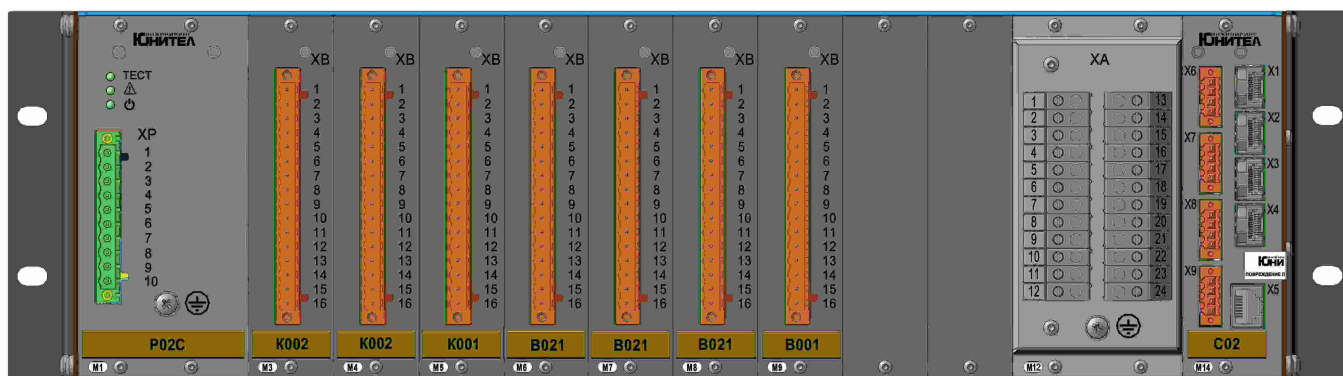
Рисунок 1.1 – Вид устройства «ЮНИТ-М319-Д3Т2» с размещением модулей по слотам (исполнение для I архитектуры)
